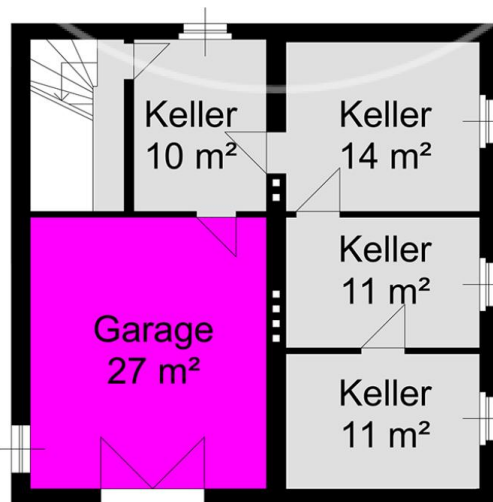
Skizze Kellergeschoss
