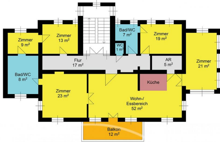
Skizze Obergeschoss
