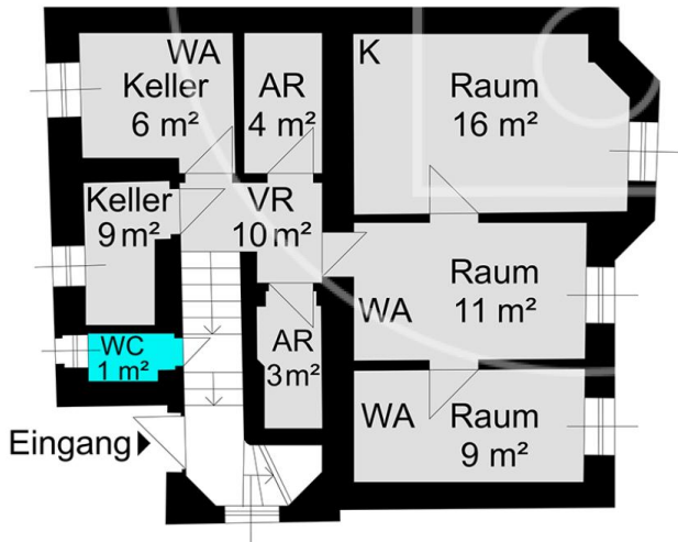
K ... Kamin VR ... Vorraum AR ... Abstellraum WA ... Wasseranschluss Skizze Souterrain
